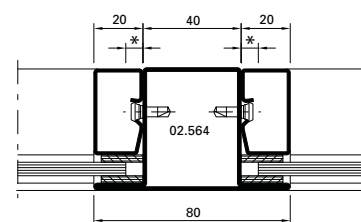
Detail příčky
