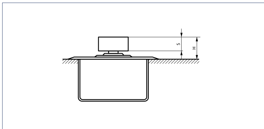
Lišta dveří model CM, C pro kyvné dveře
